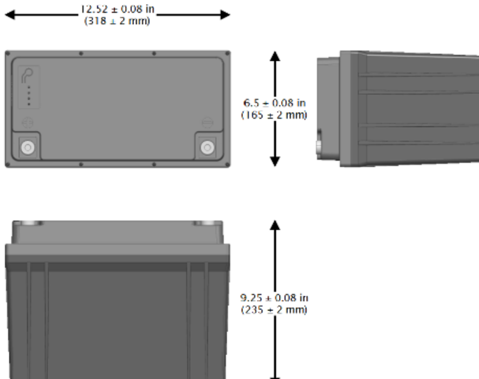
1200 HLX+ Dimensions
